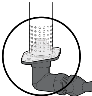
PASO 10: CONEXIÓN CORRECTA DEL QUEMADOR A LA VÁLVULA
