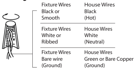
Fig.3 Wiring
