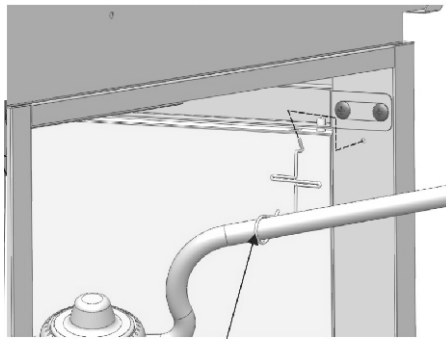
Hose hook Crochet de tuyau Gancho de la manguera
