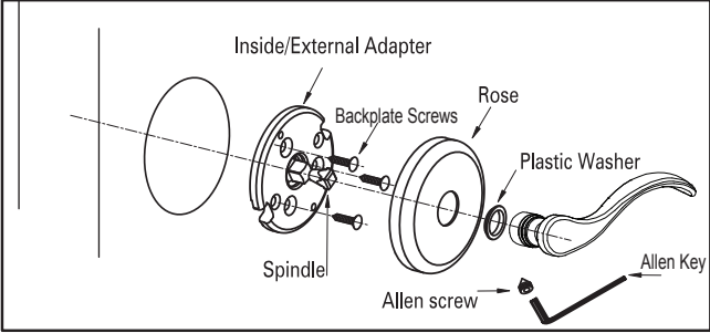
Exploded View Dummy Lockset Despiece de Cerradura Dummy Éclaté des Serrures Rossace
