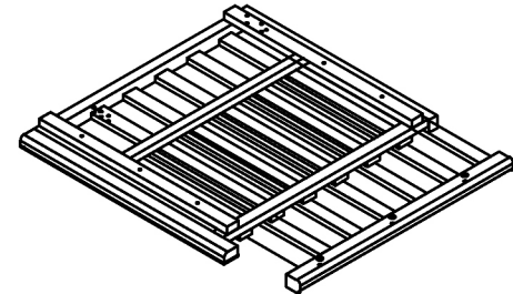
Saddle frame*2
